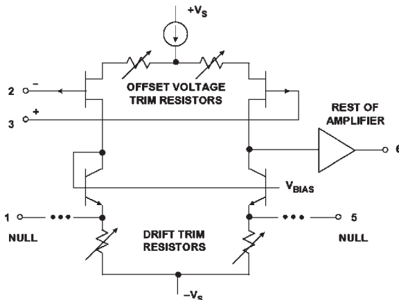
Figure 4.4.9: BiFET op amp input stage.
